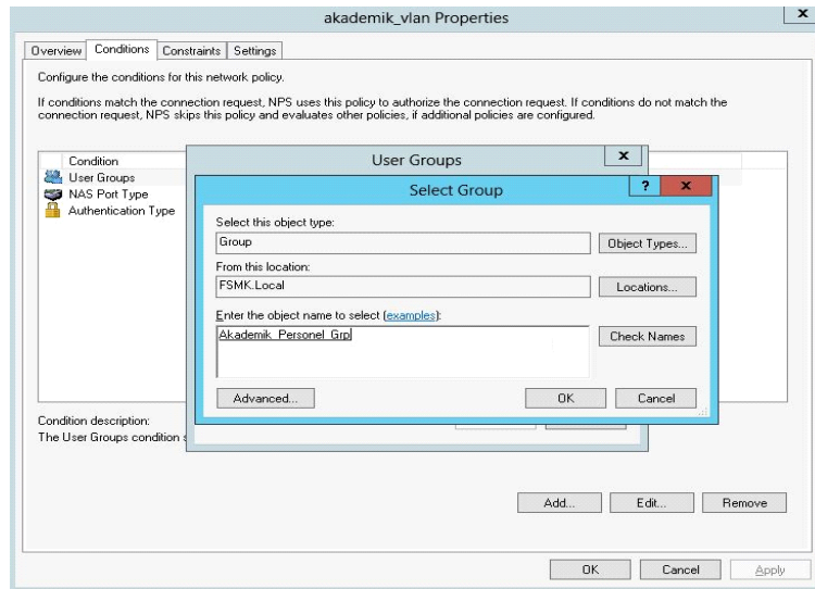
Şekil 6.42: Ağ ilkesi sunucusu 802.1x kablosuz ağ yapılandırma ekranı 9
