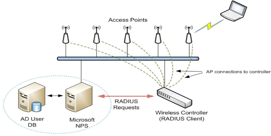
Şekil 5.5: Erişim noktası kontrolörü
