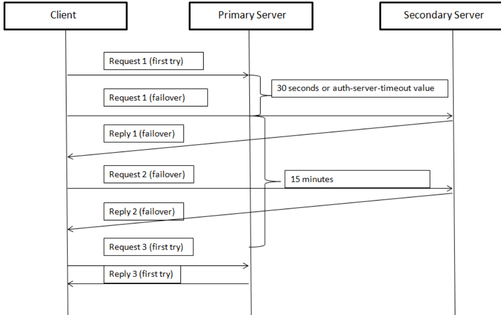
Şekil 6.67: Bağlantı hatası işlem ekranı
