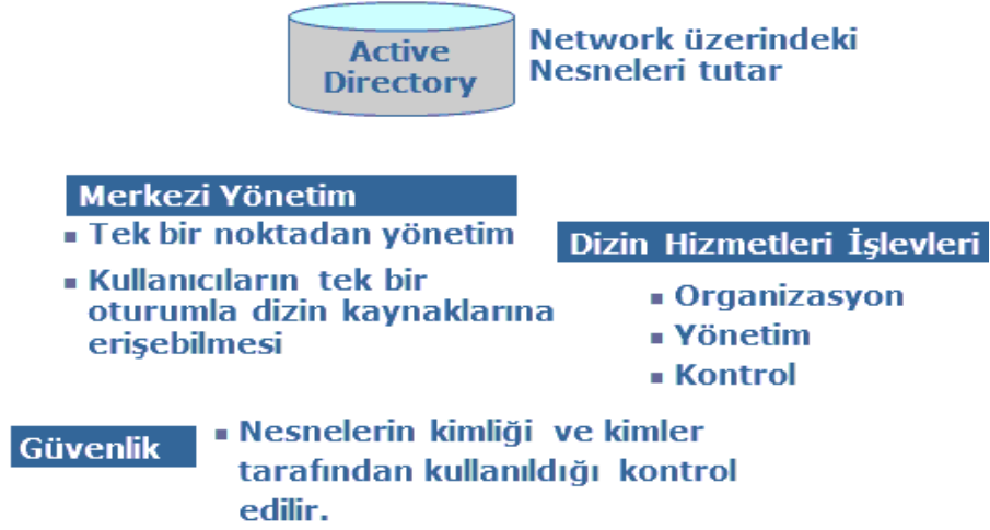
Şekil 5.2: Dizin hizmeti
