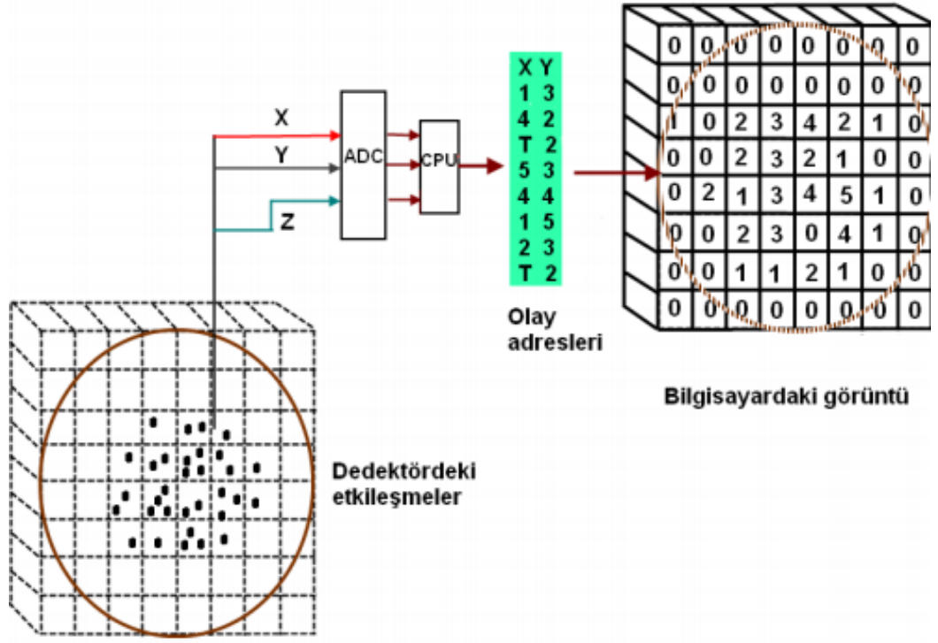
Şekil.4.10: Bilgisayarda görüntünün liste modunda toplanması
