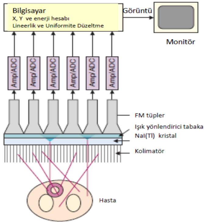
Şekil.4.4: Gama Kamera Sisteminin Bileşenleri
