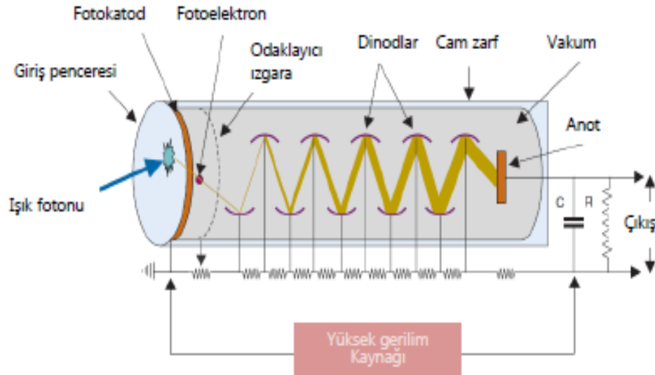
Şekil.4.6: Sintilasyon fotonlarının PMT de elektrik sinyaline dönüşmesi
