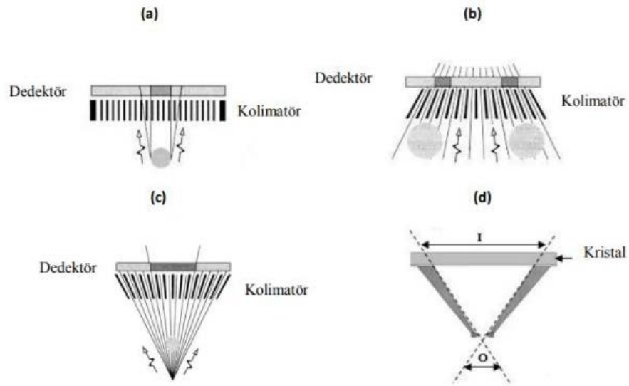
Şekil.4.5: Kolimatör Çeşitleri: a) Paralel Delikli, b) Diverjan, c) Koverjan, d) Pinhole
