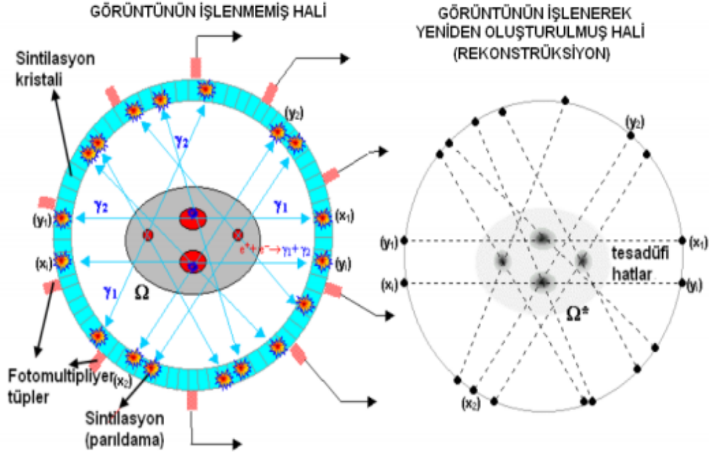
Şekil.4.14: PET cihazında görüntü oluşumu
