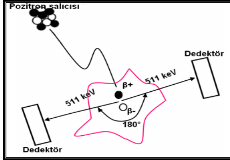
Şekil.4.12: Anhilasyon olayı
