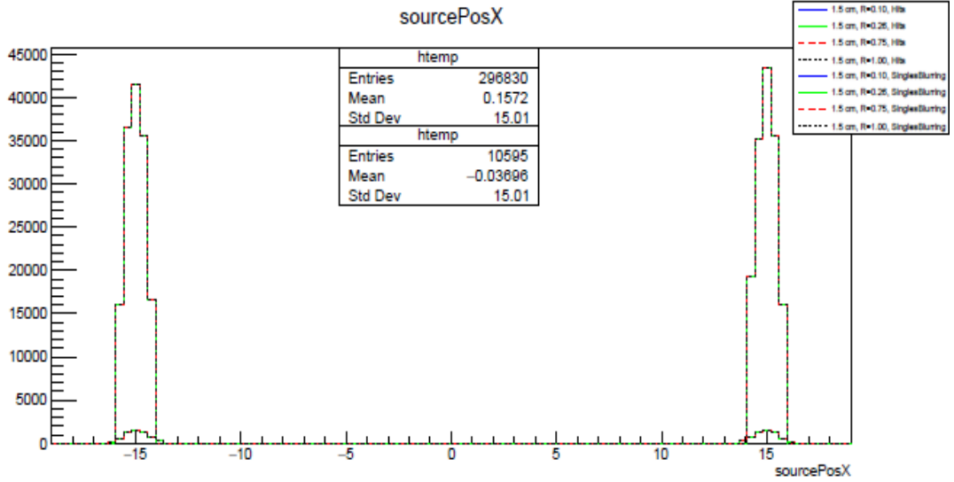
Şekil.8.9: Vuruşların ve çakışmaların verileri için (-15, + 15) mm mesafelerde yerleştirilmiş çift izotopların girişlerinin farklı çözünürlüklerde karşılaştırılması
