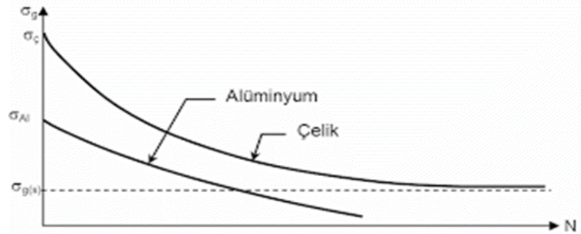
Şekil 2.3:a Wöhler-diyagramı[4].
