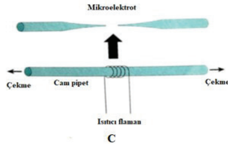
Şekil 13: A. Mikroelektrot çekici. B-C. Mikroelektrot çekici şeması (1, 11).
