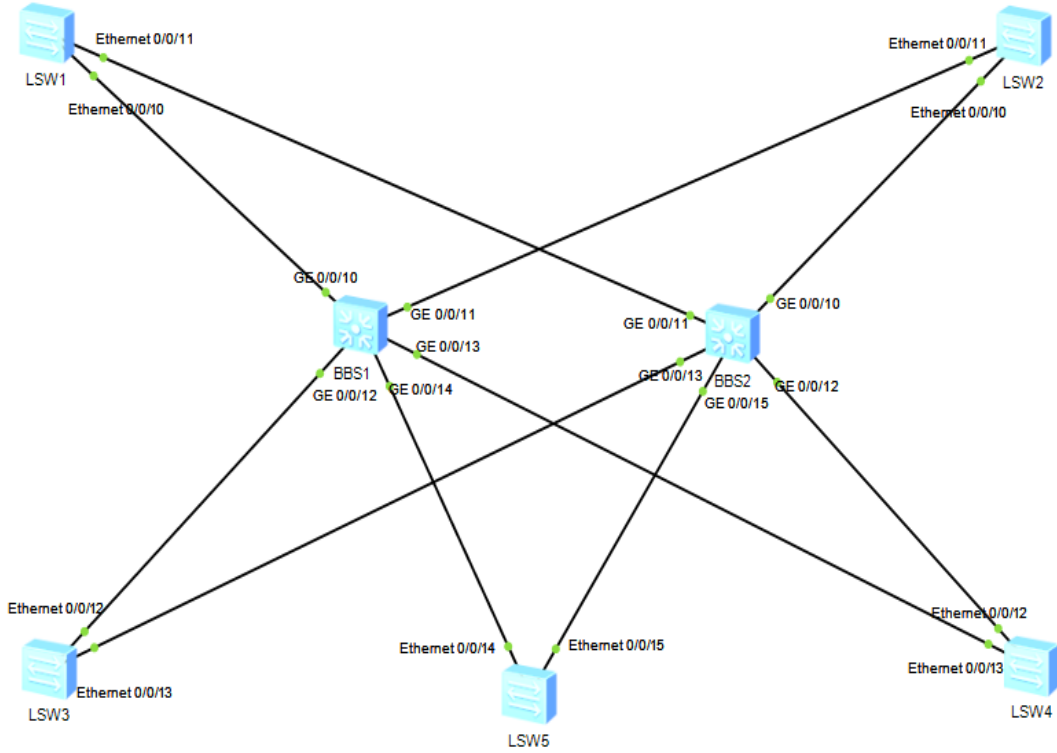
Şekil 5.5 MSTP protokolünün uygulanacağı switch'lerin haritası
