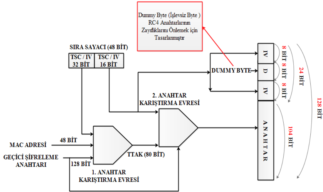
Şekil 4.10 Paketlerin şifrlenmesi için farklı anahtarların oluşturulması
