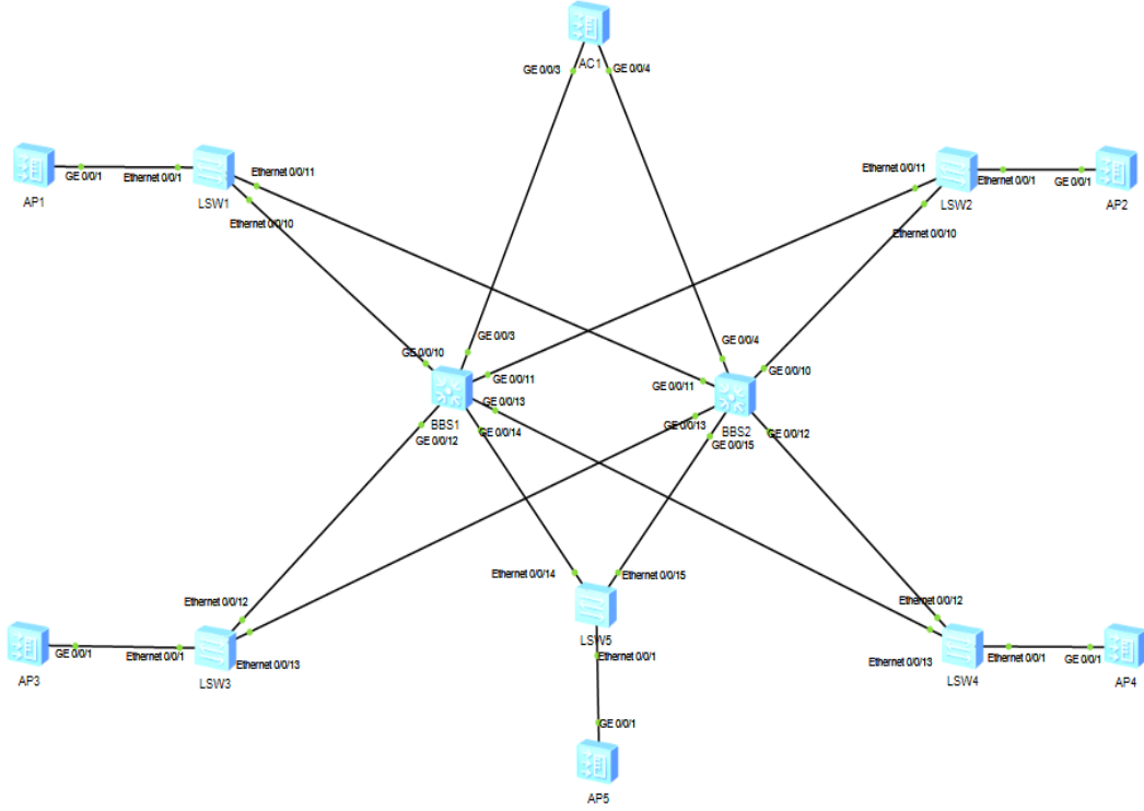
Şekil 5.6 AP'lerin eklenmiş durumu
