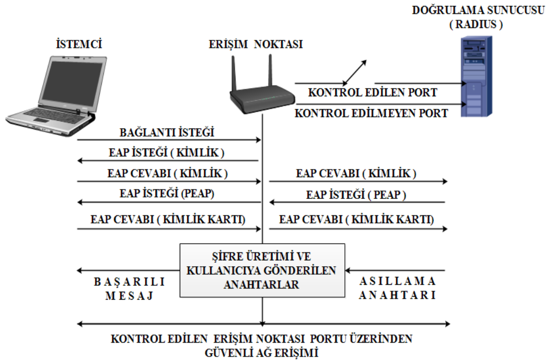
Şekil 4.9 802.1x asıllama işlemi adımları
