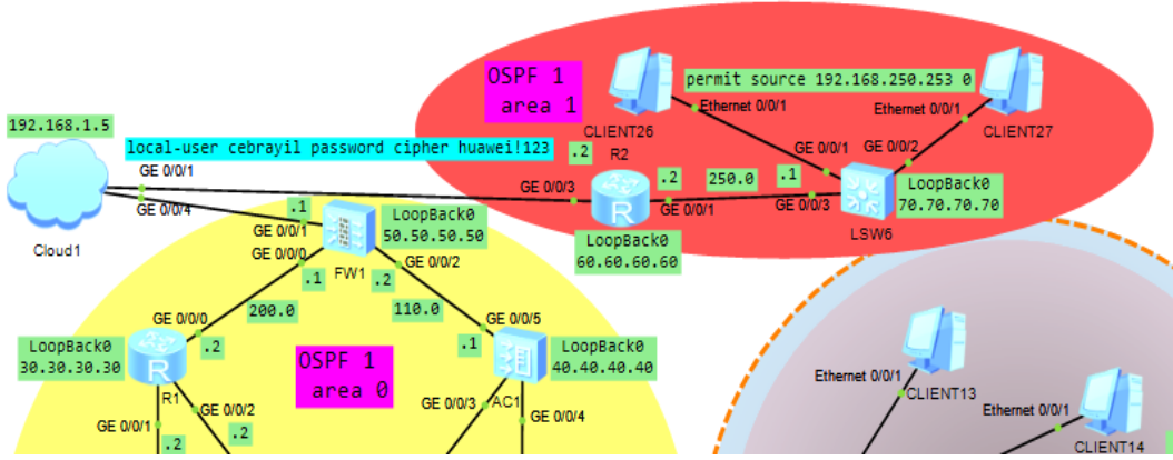
Şekil 6.5 Yeni ağın eklenmiş hali
