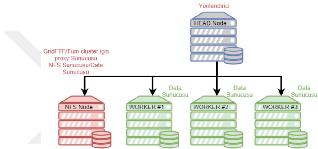
Şekil 2.3: GridFTP Yapılandırması #2
