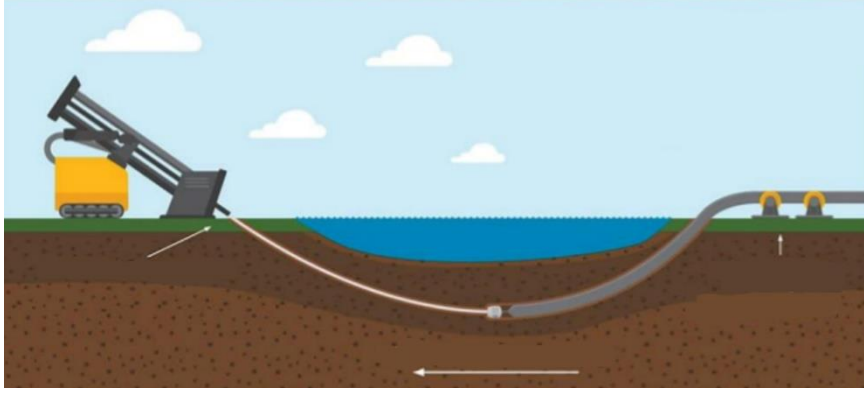
Şekil 53 Yatay Sondaj Sisteminin Çalışma Mantığı (Coosbay.org, 2019)
