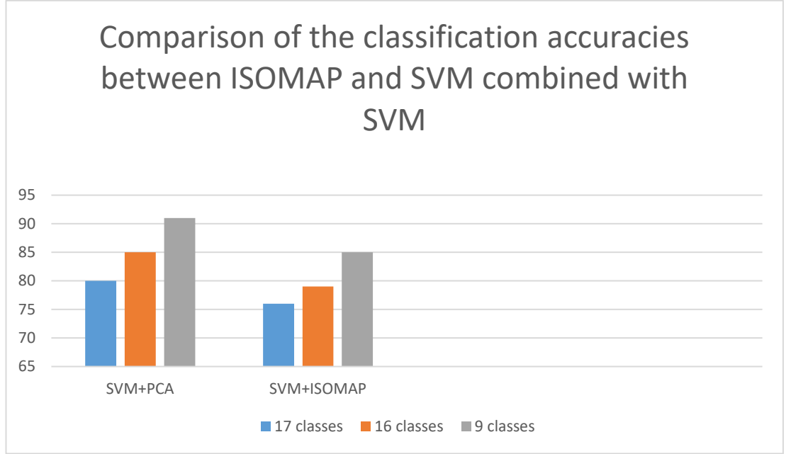
Şekil 4.59: PCA-SVM ve ISOMAP-SVM yöntemlerinin karşılaştırılması
