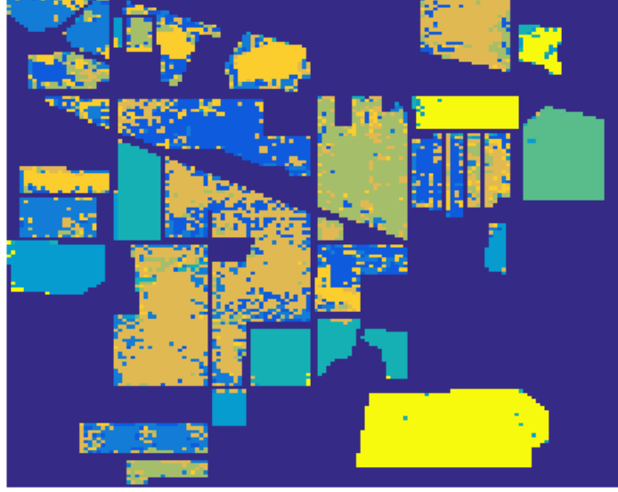
Şekil 4.35: 9 sınıflı durumda ilk 50 ISOMAP özneliği için KNN sınıflandırma sonucu
