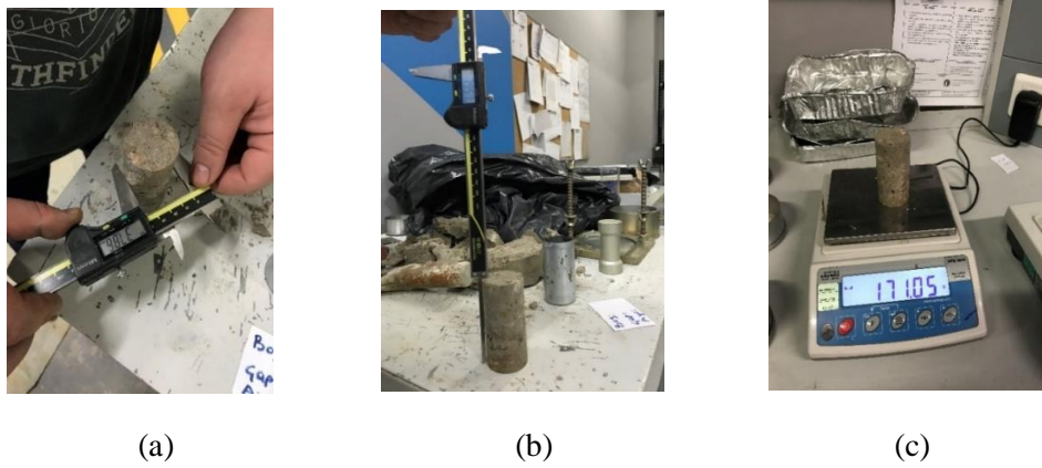
Şekil 4.26: Üç eksenli basınç deney numunesinin çapının, boyunun ve ağırlığının ölçülmesi
