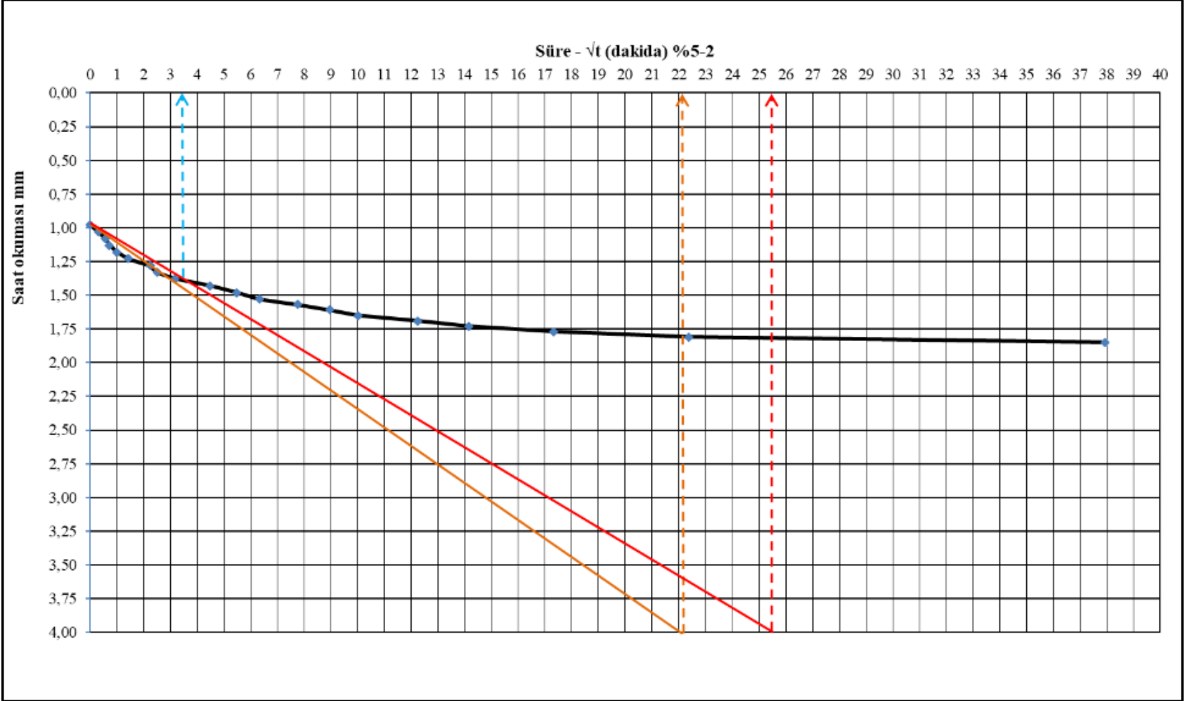
Şekil B.2: %5 çimento katkılı kumlu kil 2.halka konsolidasyon deneyi oturma-karekök zaman grafiği
