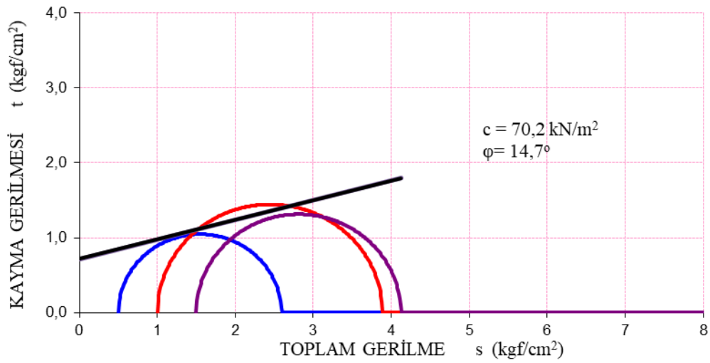
Şekil 5.6: %10 çimento katkılı 1.set üç eksenli basınç deneyinden elde edilen mohr daireleri
