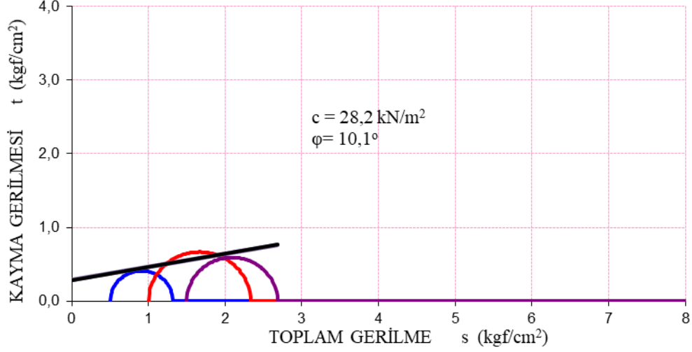
řekil 5.12: %20 imento katkılı 1.set üç eksenli basın deneyinden elde edilen mohr daireleri
