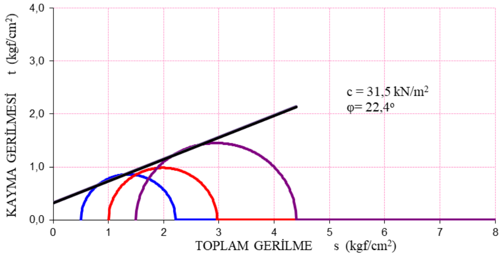
řekil 5.13: %20 imento katkılı 2.set üç eksenli basın deneyinden elde edilen mohr daireleri
