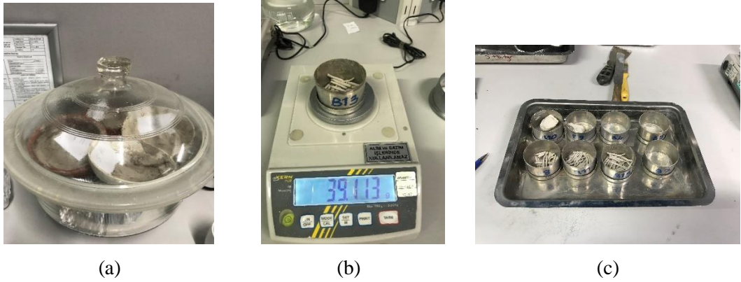
Şekil 4.15: Plastik limit deneyi yapım aşamaları
