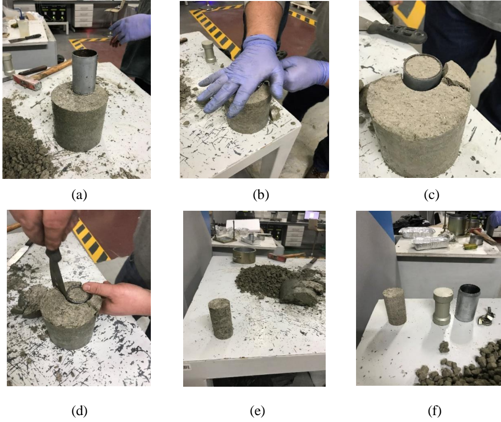
Şekil 4.25: Üç eksenli basınç deney numunelerinin hazırlanması
