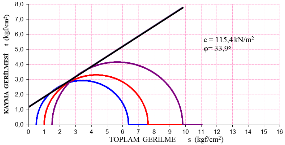
Şekil 5.18: 7 günlük %5 çimento katkılı 2.set üç eksenli basınç deneyinden elde edilen mohr daireleri
