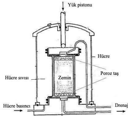
Şekil 2.3: Üç aksel basıncı deneyi (Önalp, 2007)
