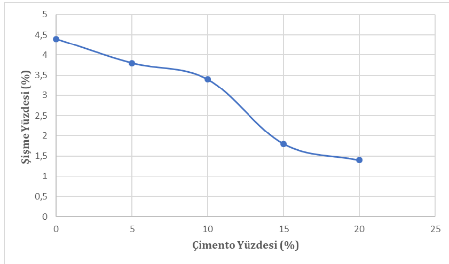
Şekil 5.30: Çimento yüzdesine bağlı numune şişme yüzdesi değerlerinin grafikte gösterimi
