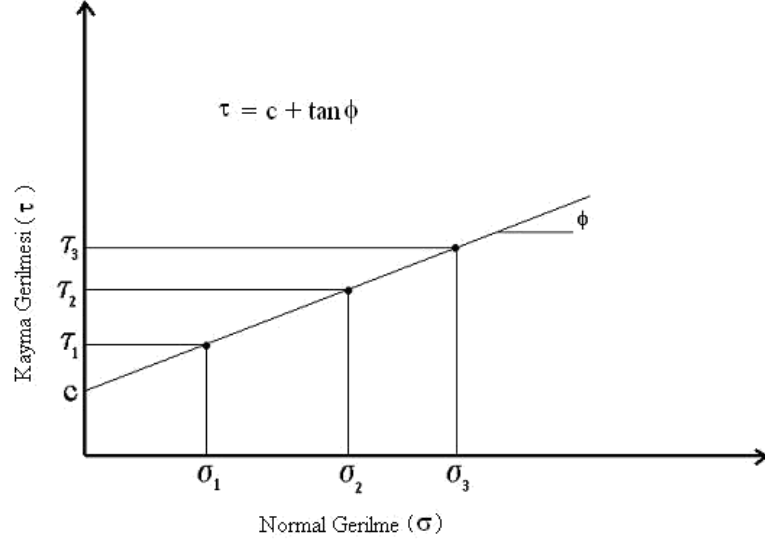
Şekil 2.1: Coulomb göçme zarfı (Özaydın 2010)
