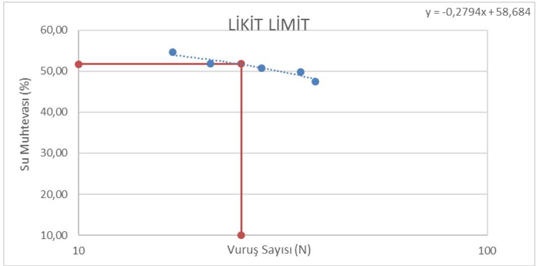
Şekil 4.21: 3. deney sonucu likit limit değeri
