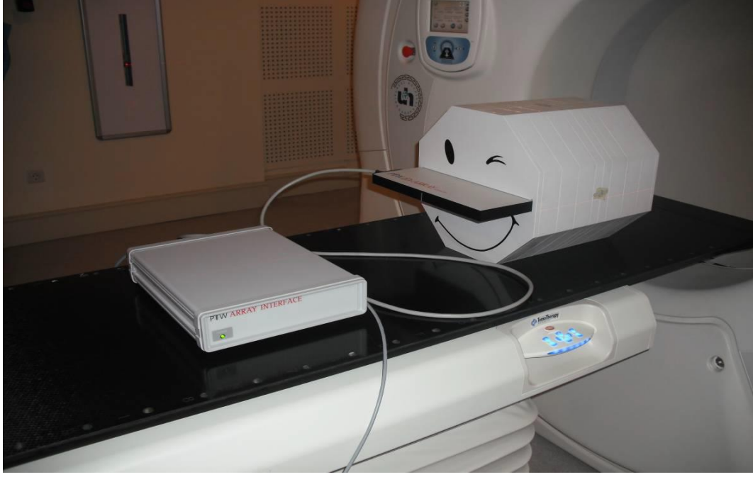
Şekil 7.7: 2D Array 729 iyon odası Octavius fantom setubü
